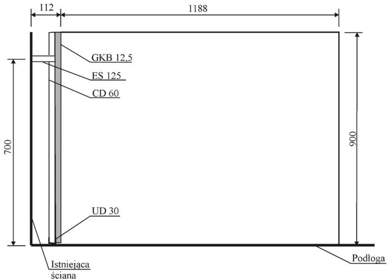
PRZEKRÓJ A-A
