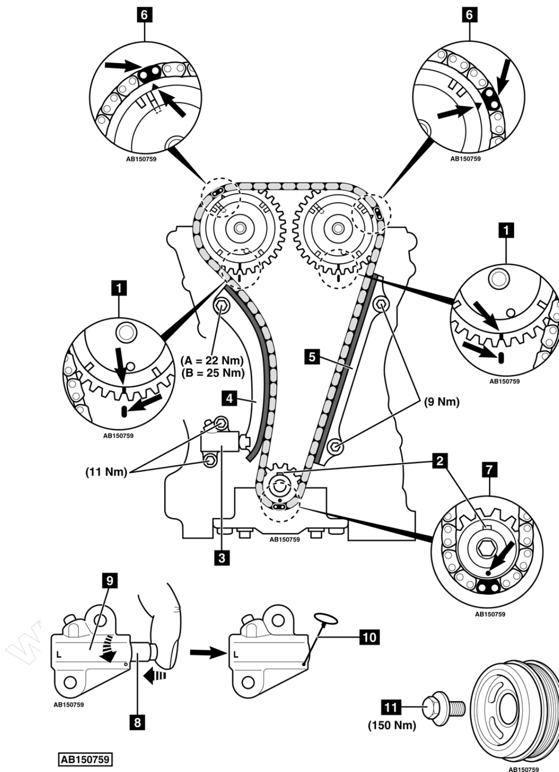
Rysunek 2. Schemat napędu rozrządu
