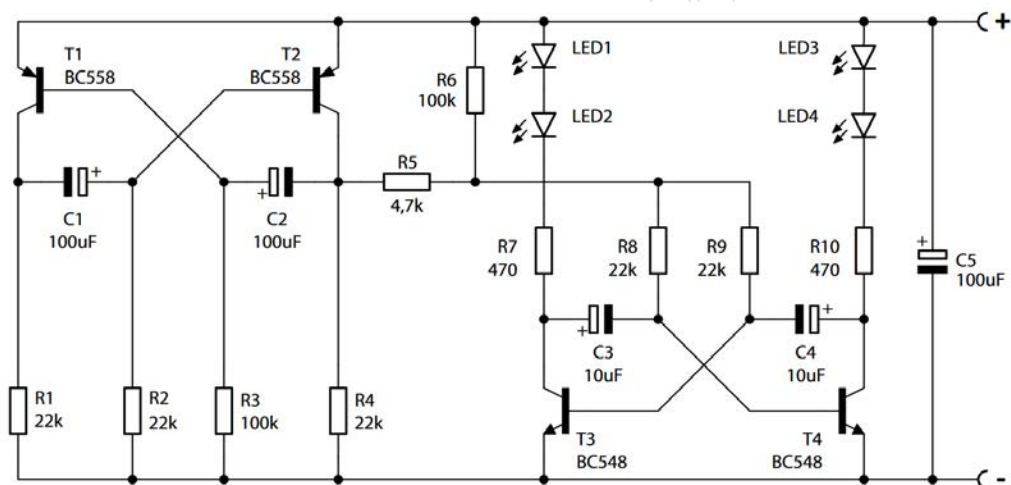
Schemat ideowy
