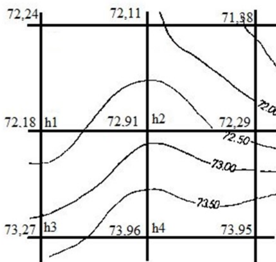
Rys. 2 Siatka kwadratów do obliczenia mas ziemnych
