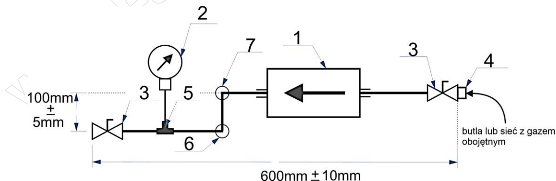
Rysunek 1. Schemat zespołu filtra odwadniacza
