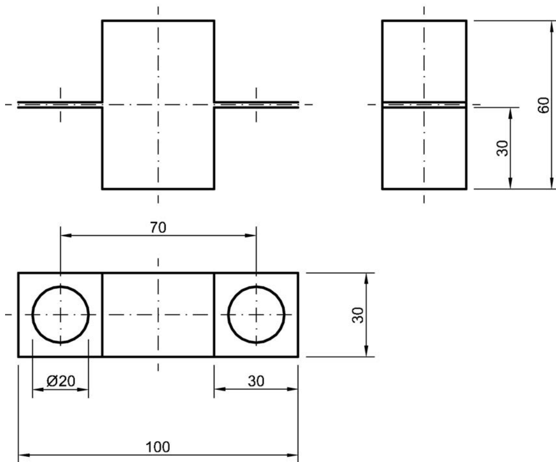
Rysunek 1. Obejma
