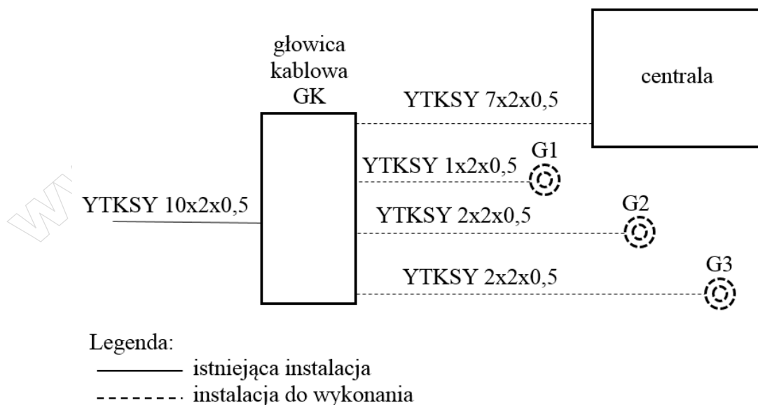
Rysunek 1. Schemat elektryczny instalacji
