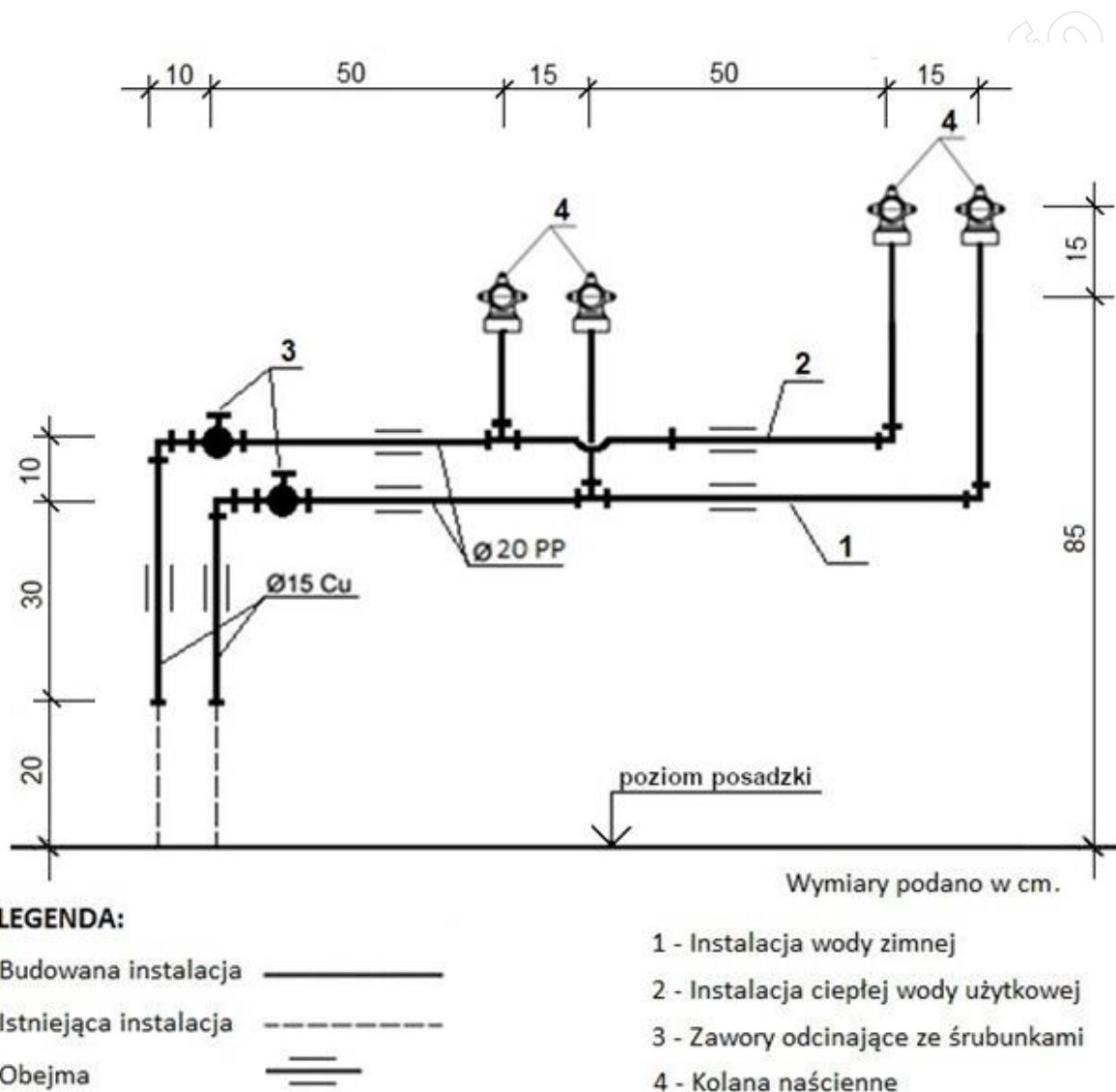
Rysunek 1. Instalacja wody zimnej i ciepłej wody użytkowej – fragment
