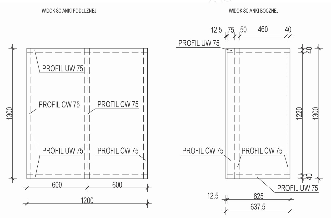
Rusunek nr 1. Konstrukcja z profili.
