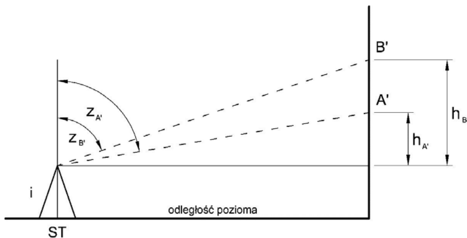
Rysunek 2. Rzut pionowy położenia punktów kontrolowanych A' i B'
