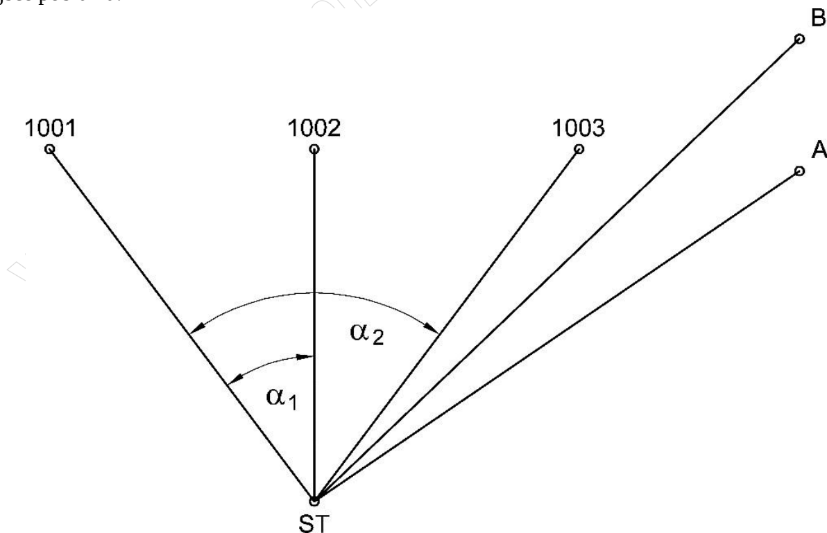
Rysunek 1. Szkic rozmieszczenia punktów kontrolowanych A' i B' względem punktów osnowy 1001, 1002, 1003 oraz ST
