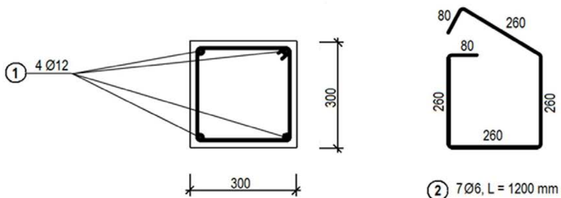
Rysunek konstrukcyjny fragmentu słupa żelbetowego
