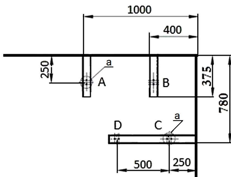
Rysunek 3. Rozmieszczenie kątowników w narożniku - wymiary podane w mm
