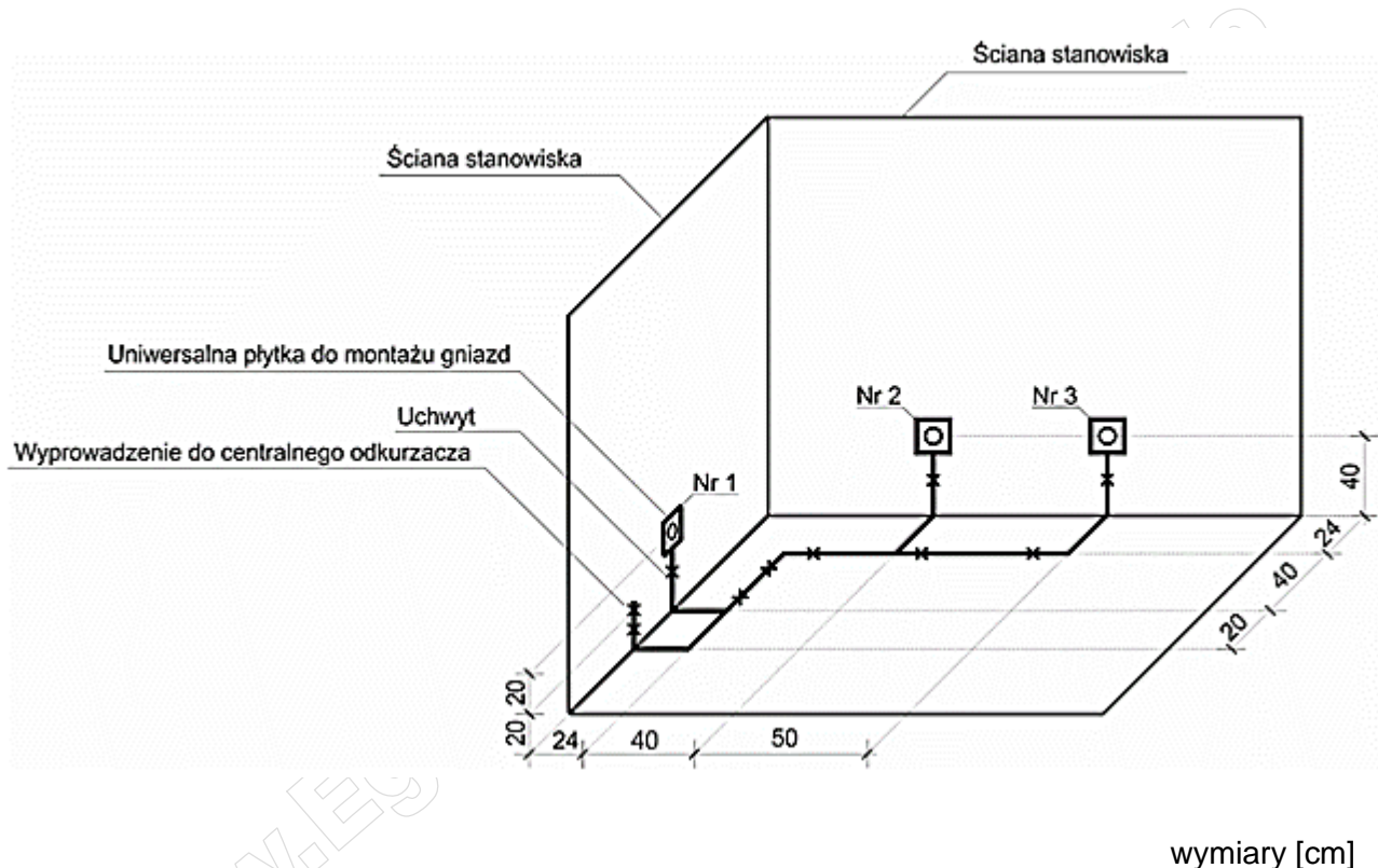
Rysunek 1. Widok fragmentu instalacji centralnego odkurzacza
