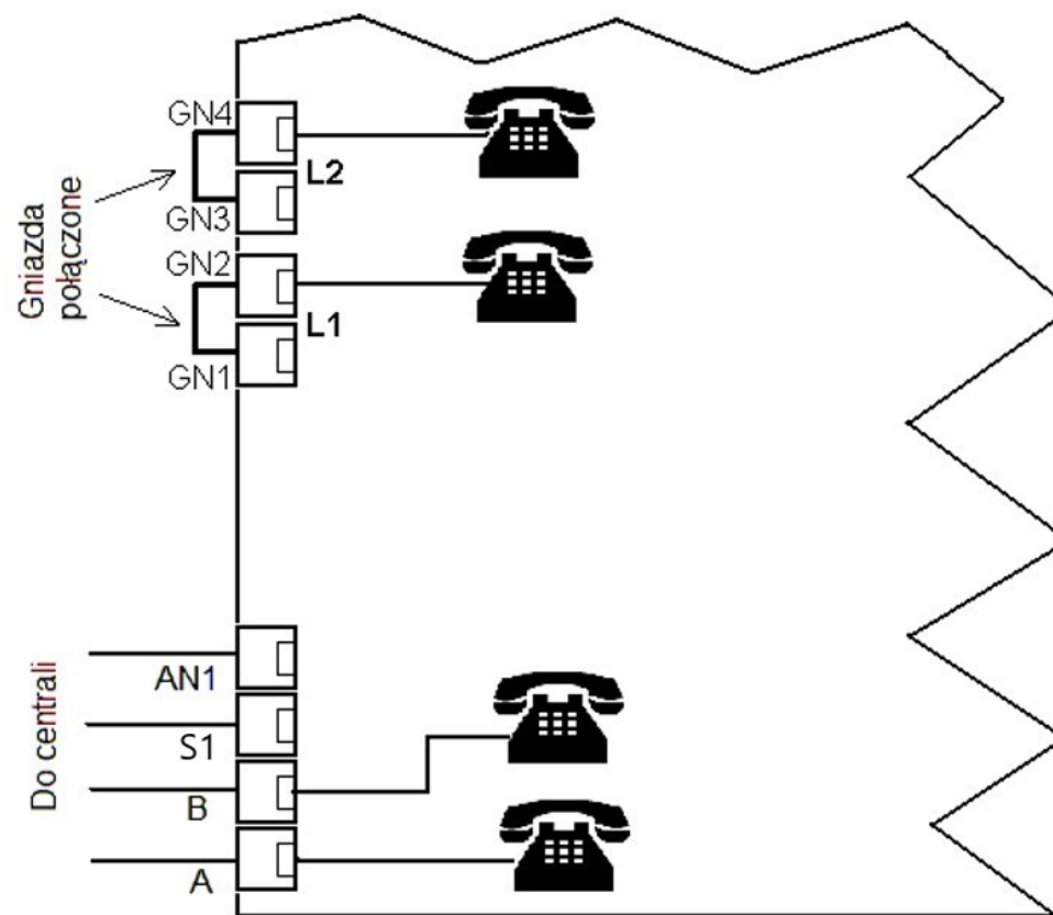
Rozmieszczenie gniazd przyłączeniowych na stanowisku egzaminacyjnym
