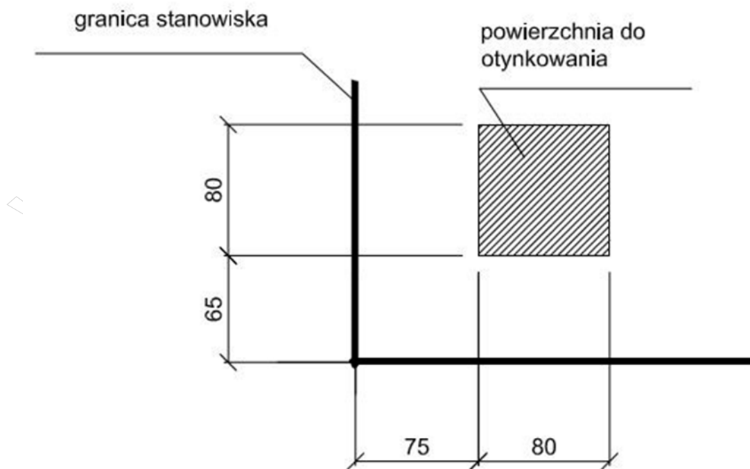
Rysunek 4. Usytuowanie tynku cienkowarstwowego mozaikowego na ścianie
