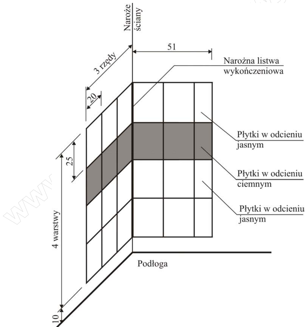
Rysunek 1. Okładzina ścienna w narożu
