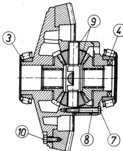
Rysunek 9. Mechanizm różnicowy
