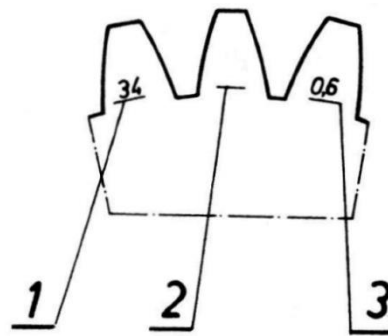
Rysunek 3. Oznakowanie czola zębów wałka atakującego
