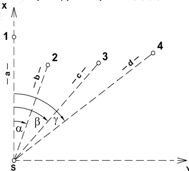
Rzut poziomy położenia punktów S, 1, 2, 3, 4
