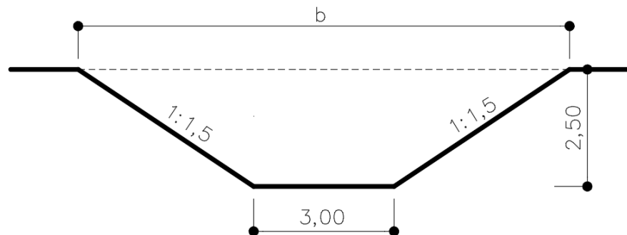
Rysunek 1. Przekrój poprzeczny wykopu
