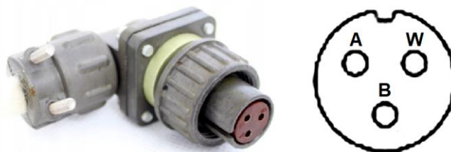
Rysunek 7. Złącze wtykowe SzP-3 stosowane do podłączenia instalacji elektrycznej radiostacji XCOM-760 do zasilacza akumulatorowego
