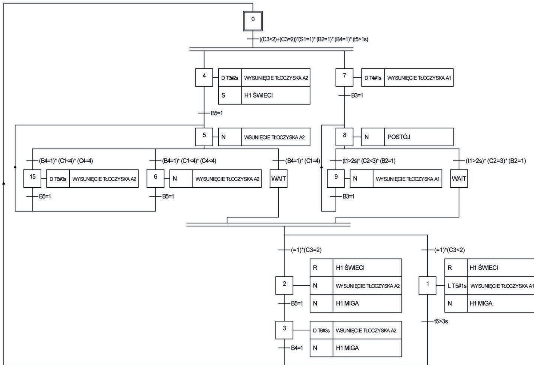
Rys. 4. Algorytm działania układu elektropneumatycznego
