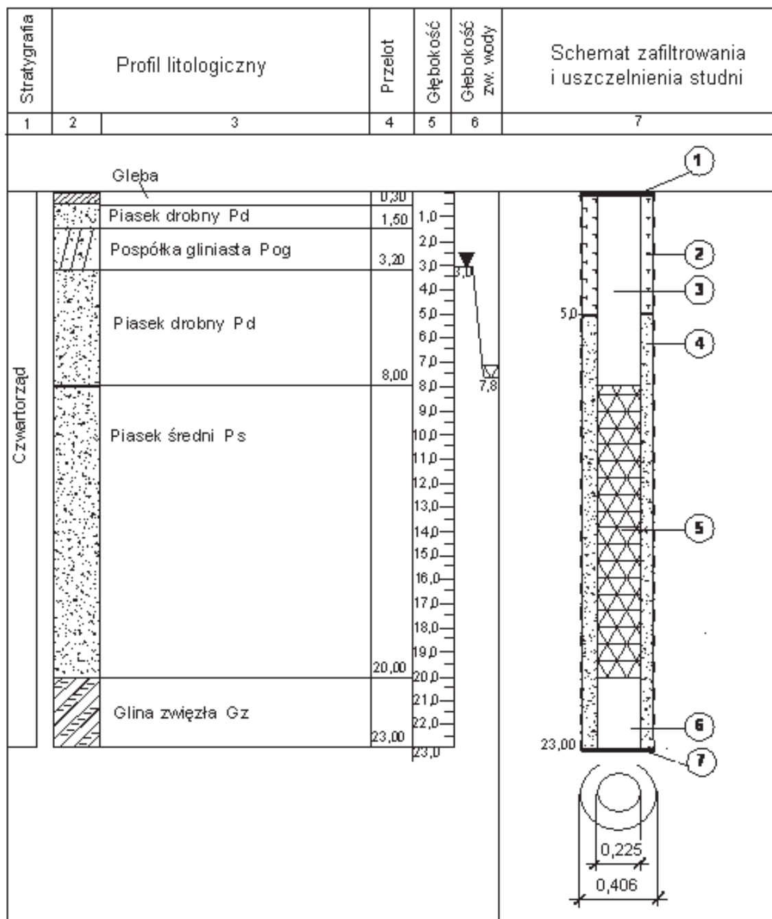
Rysunek 1. Profil litologiczny i schemat zafiltrowanego otworu studziennego wraz z warstwami jego uszczelnienia
