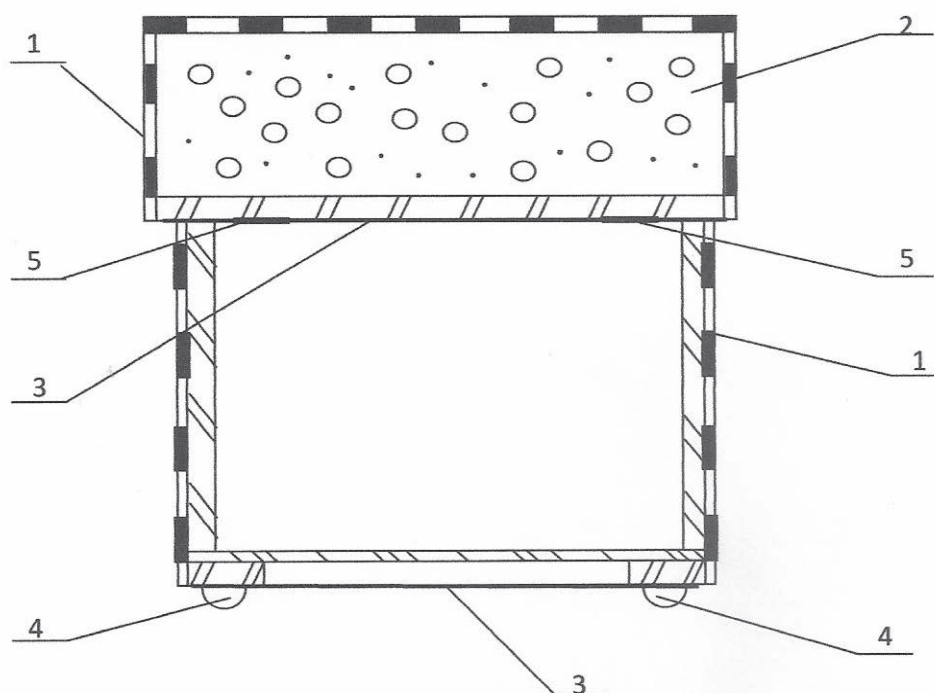
Rys. 1 – przekrój pufu.
