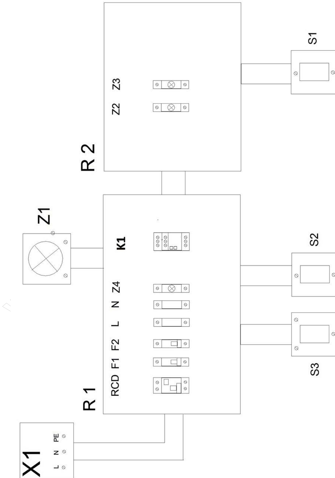
Rys. 3. Schemat montażowy instalacji elektrycznej (do uzupełnienia)
