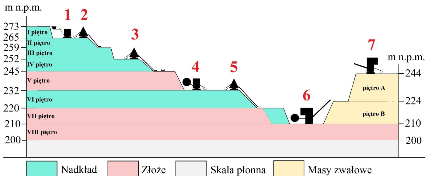
Rysunek. Profil geologiczno-górnictwa wyrobiska wraz ze schematem pracy maszyn
