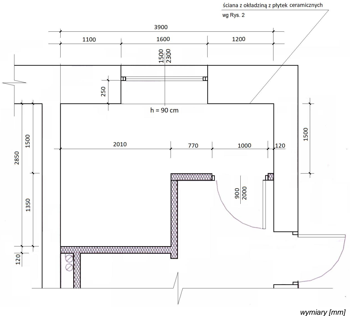
Rysunek 1. Rzut łazienki
