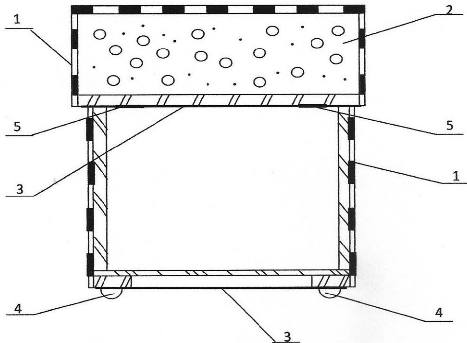
Rys. 1 – przekrój pufu
