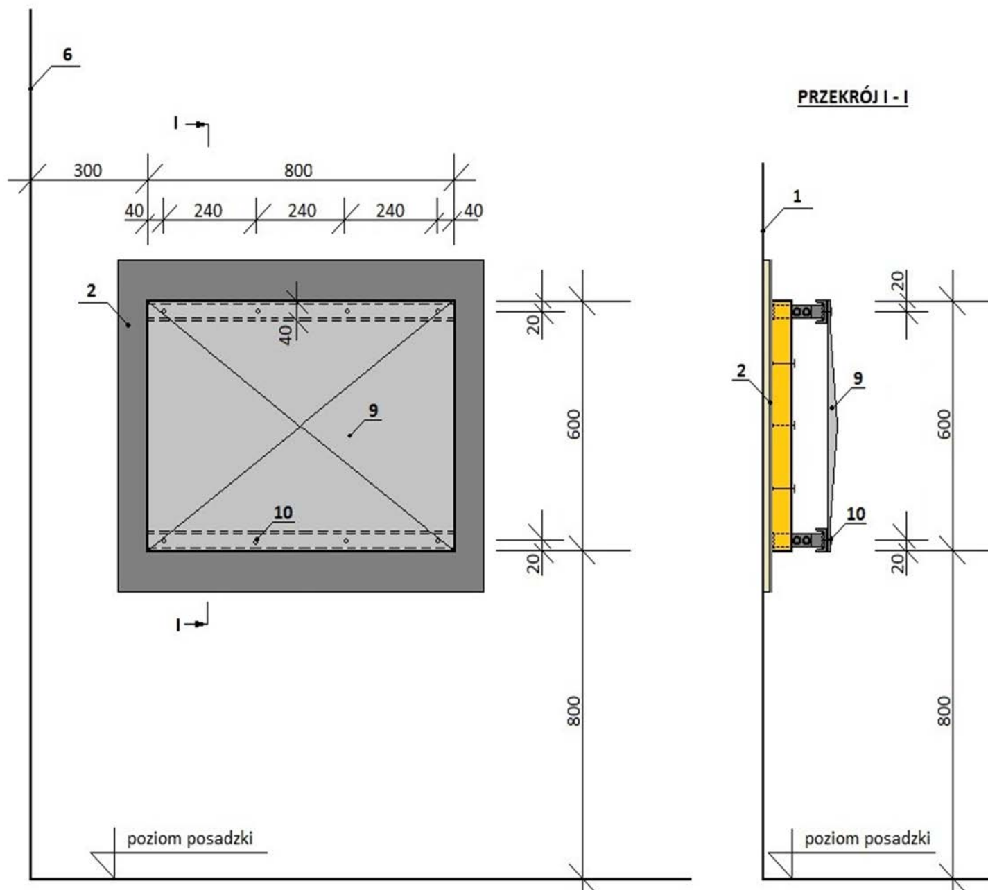
Rysunek 3. Widok i przekrój płaszcza ochronnego izolacji z blachy płaskiej kopertowanej
