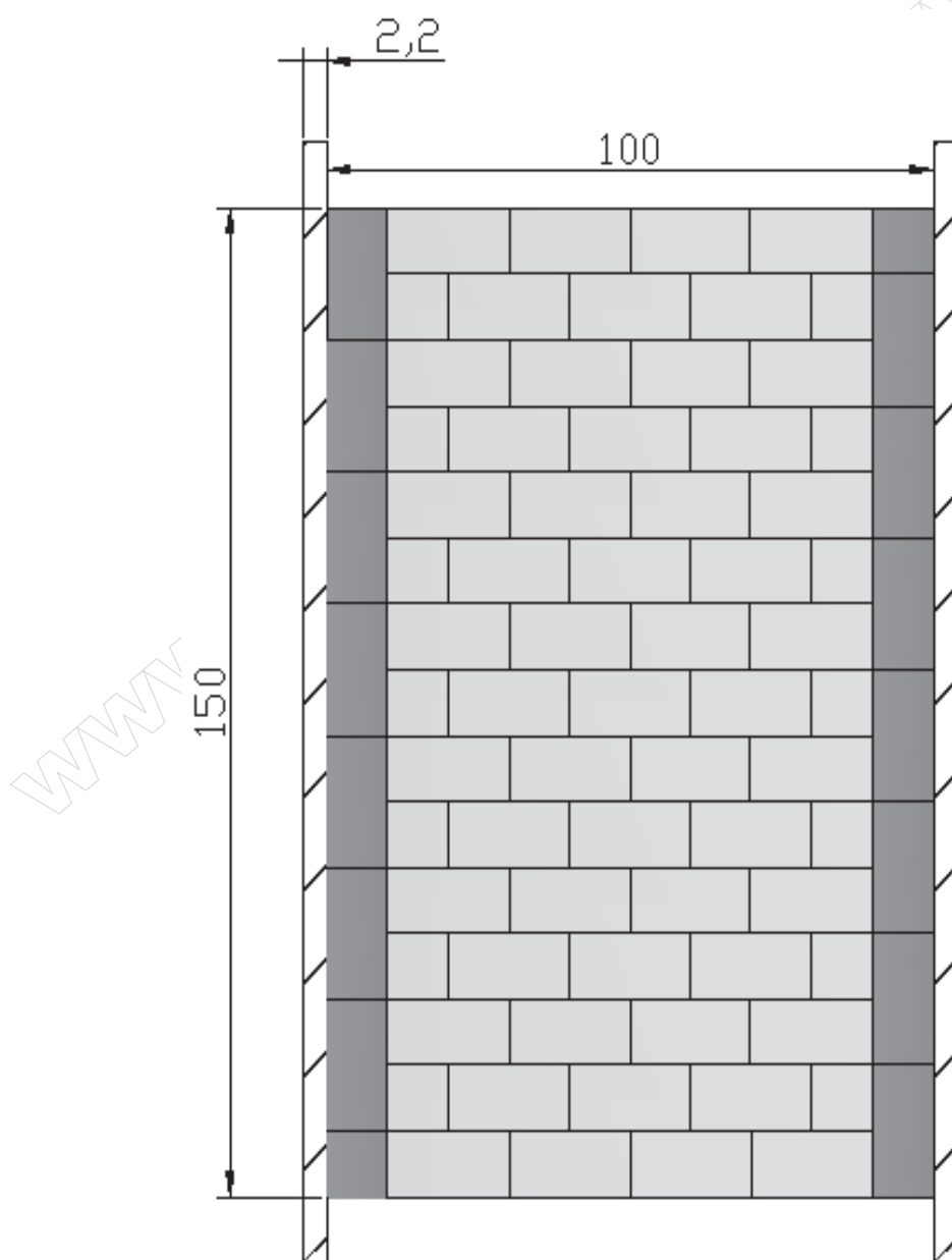
Rysunek nr 1. Rzut poziomy chodnika [wymiary w cm]
