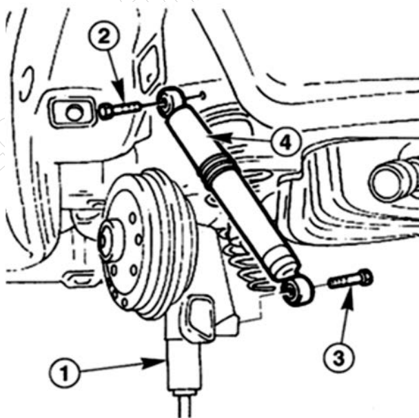
Rys 2. Zamocowanie amortyzatora
