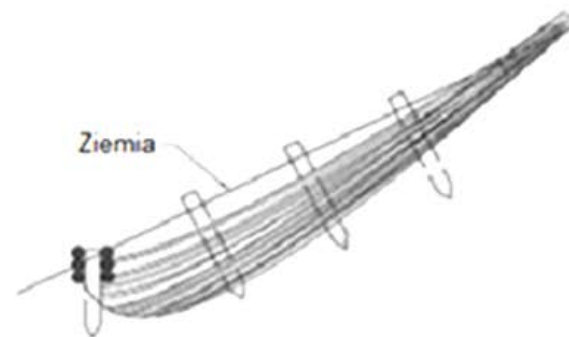
Etap 4 - przykrycie ziemią materaca faszynowego
