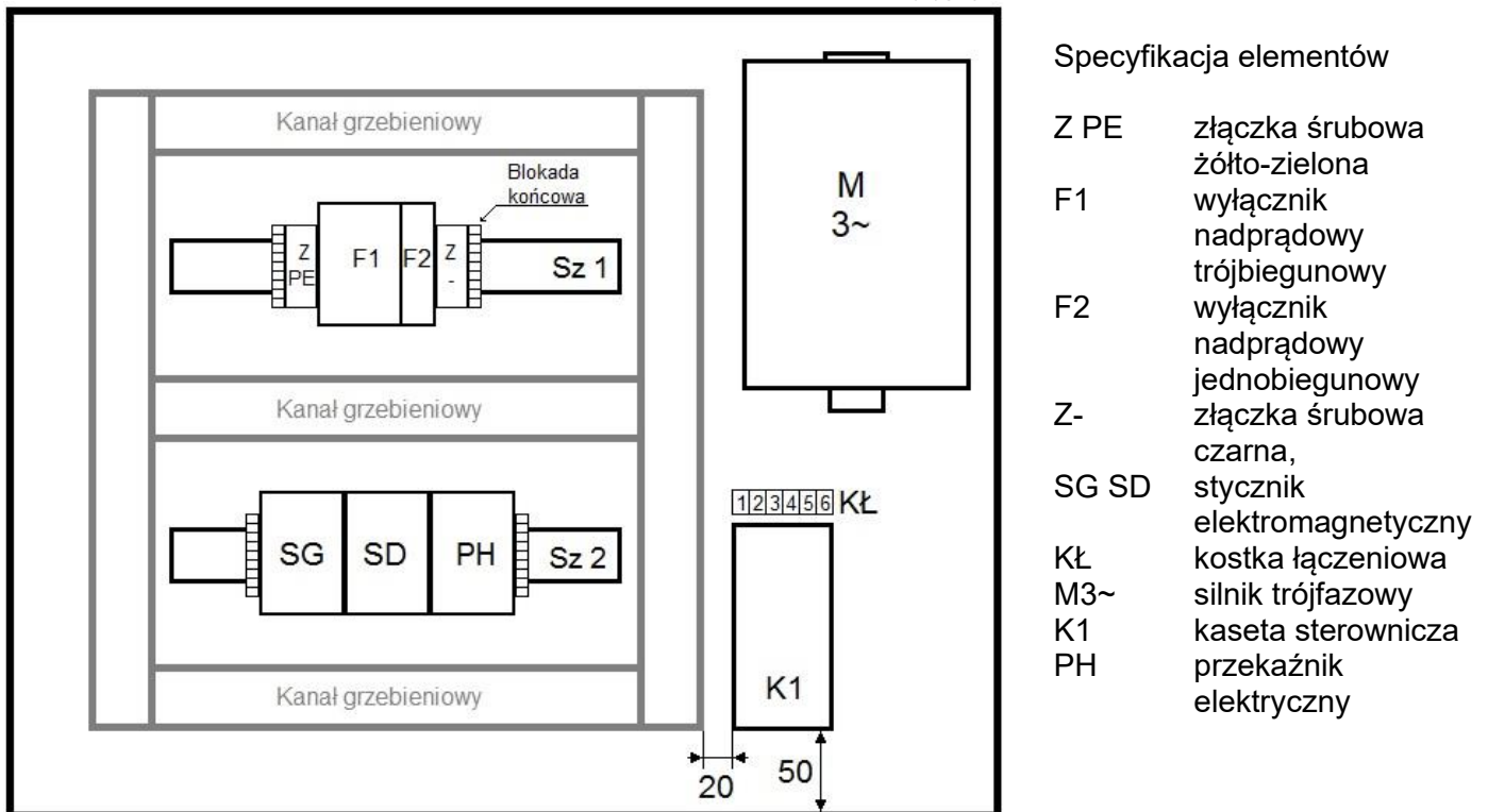
Rysunek 1. Rozmieszczenie elementów na płycie montażowej
