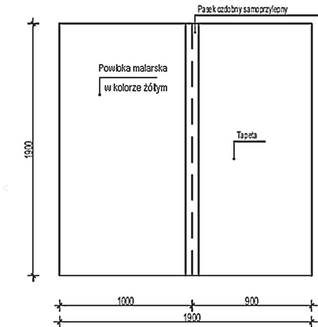
Widok ściany
