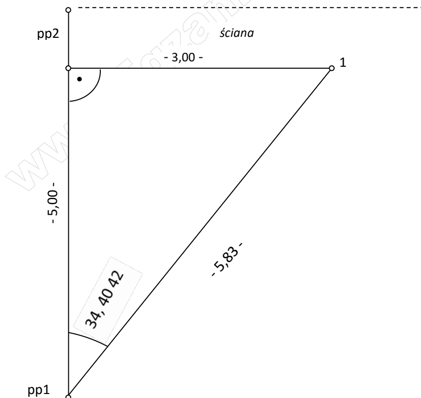
Rysunek 1. Szkic rozmieszczenia punktów – rzut poziomy
