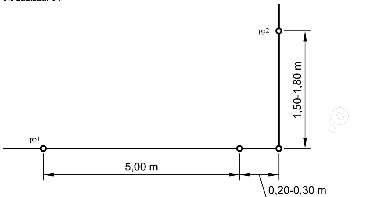
Rysunek 2. Szkic rozmieszczenia punktów – przekrój pionowy
