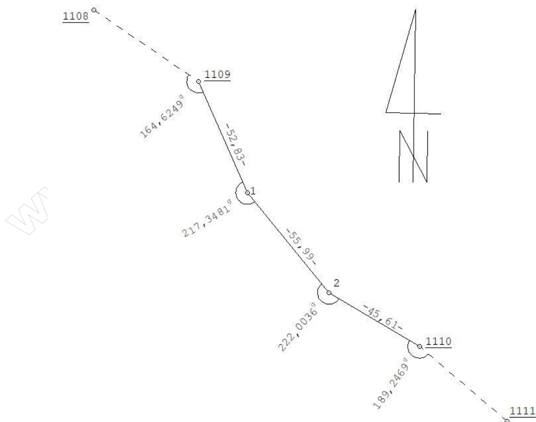
Rysunek 2. Szkic z pomiaru sytuacyjnego ciągu poligonowego
