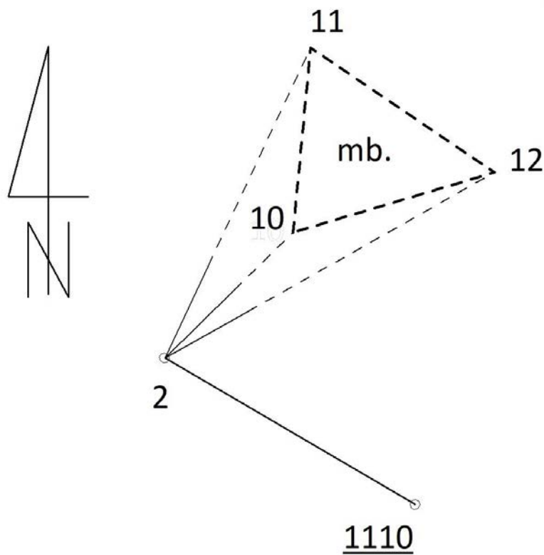
Rysunek 1. Szkic sytuacyjny położenia obszaru utwardzonego masą bitumiczną
