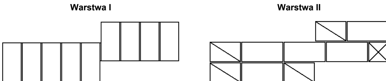
Rysunek 2. Układ cegieł w pierwszej i drugiej warstwie muru (rzuty)
