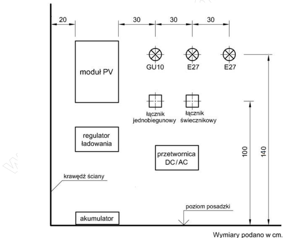
Rysunek 1. Schemat rozmieszczenia elementów instalacji
