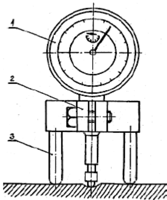
Rys. 13.2. Czujnik z podstawą do pomiaru głębokości wgłębień na dźwigarze łopaty 1–czujnik, 2–ściągacz; 3–nóżka
