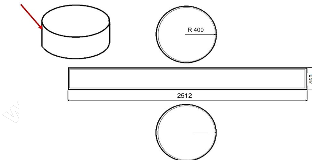
Rysunek 1. Poszewka wewnętrzna pufu kibica
