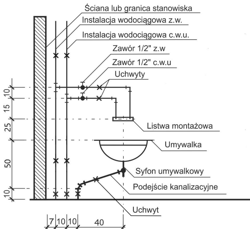
Rysunek 1. Widok instalacji wodociągowej i kanalizacyjnej
