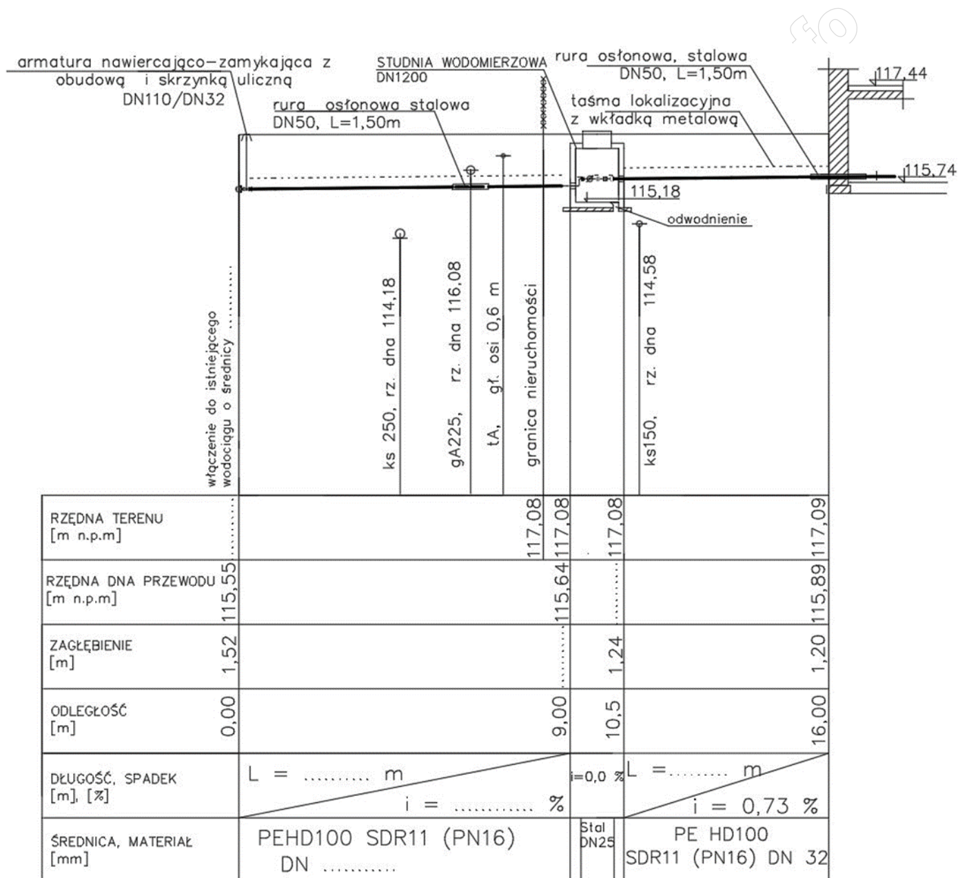
Rysunek 2. Profil przyłącza wodociągowego
