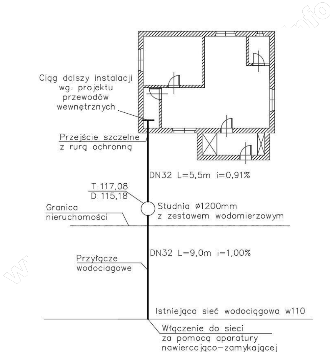
Rysunek 1. Schemat przyłącza wodociągowego
