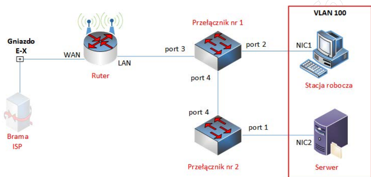
Rys. Schemat połączenia urządzeń sieciowych
