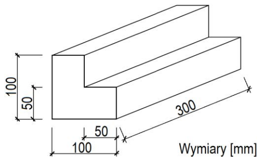
Rysunek poglądowy elementu betonowego
