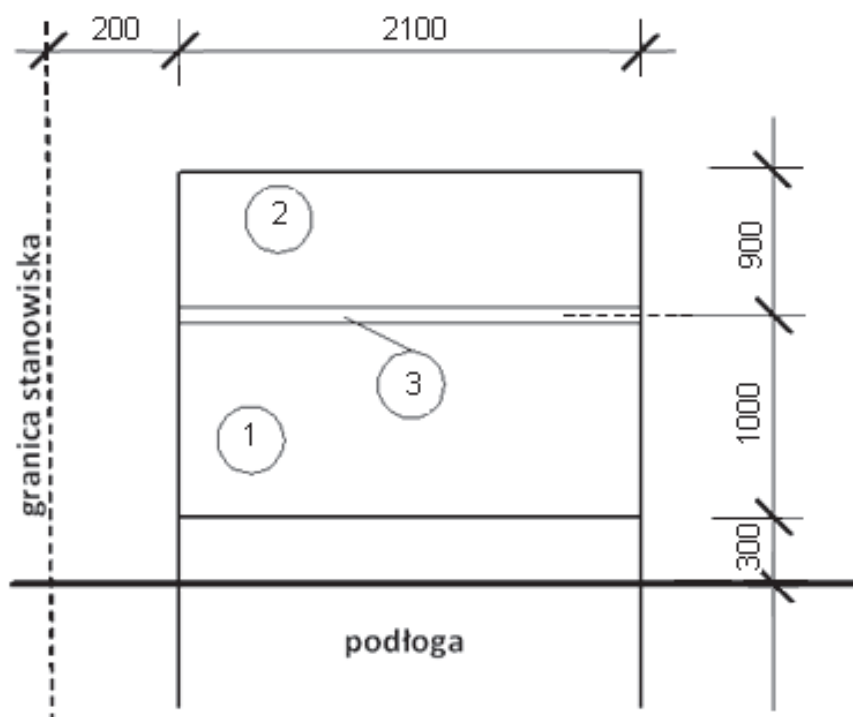
Widok ściany
