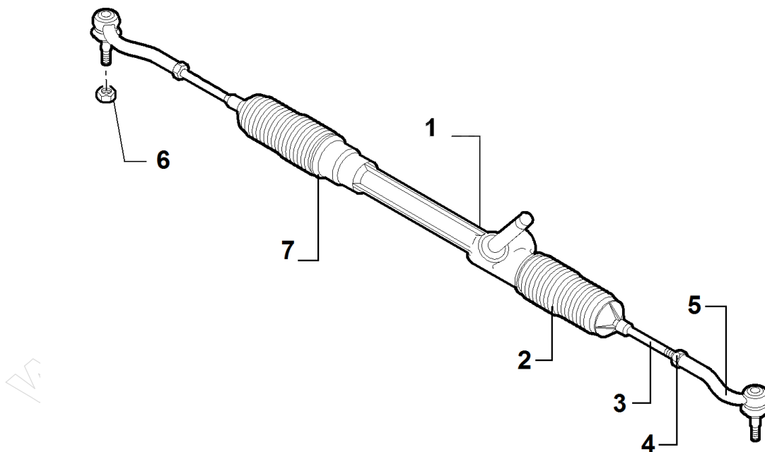
Rys. 2. Elementy układu kierowniczego Fiat 500C
