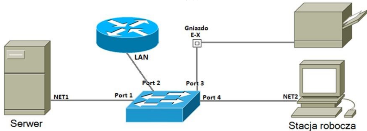
Schemat połączenia urządzeń
