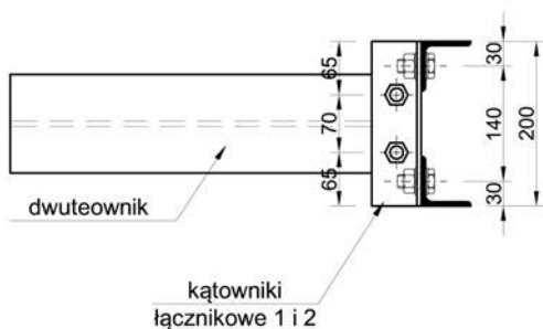
WIDOK BOCZNY:
