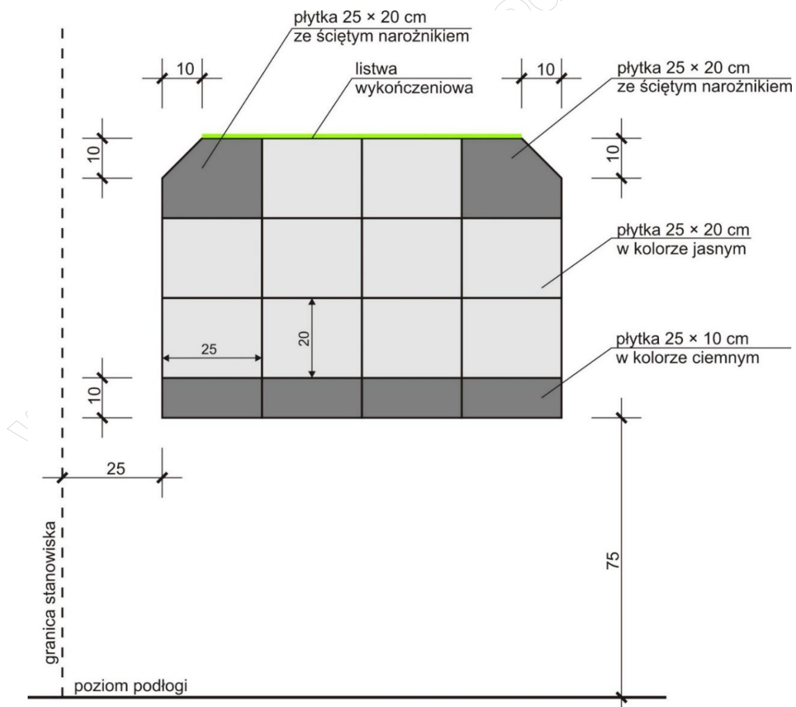
Widok okładziny z płytek ceramicznych
