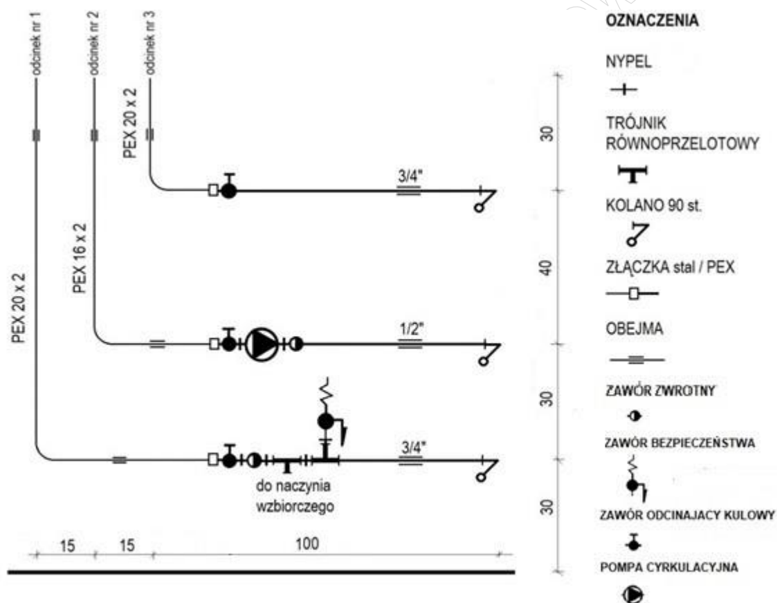
Rysunek nr 1. Schemat doprowadzenia przewodów instalacji zimnej i ciepłej wody oraz cyrkulacji do zasobnika c.w.u. (wymiały w cm)
