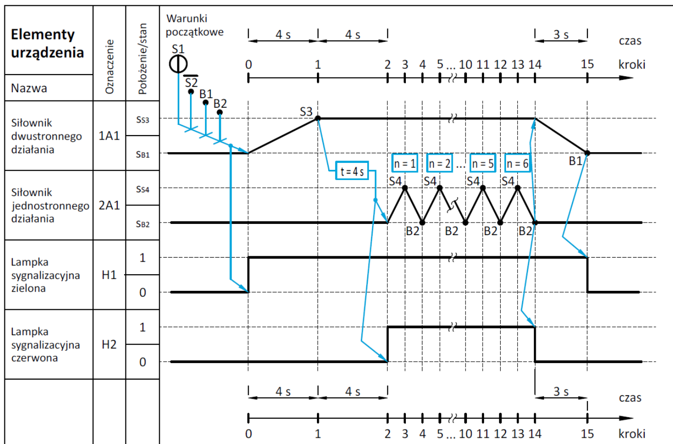
Rysunek 2. Cyklogram pracy napędu mechatronicznego*
